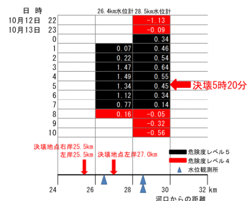
図1 堤防決壊地点の河川水位情報推移
